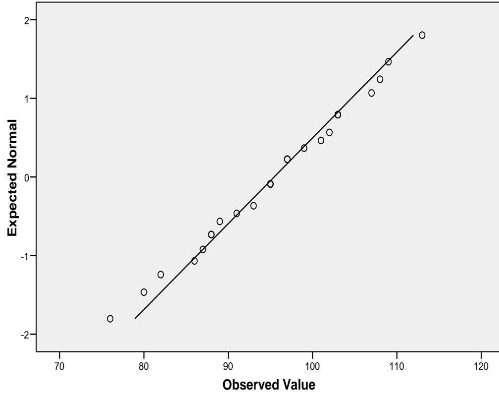
Normal Q-Q Plot of motivasi_belajar_PAI
