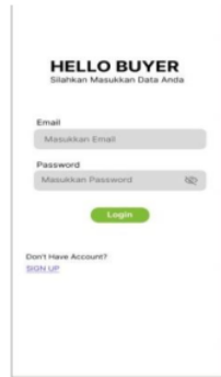
Gambar 6 Tampilan Login
