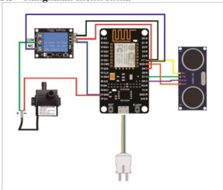
Gambar 7. Rangkaian Elektronika
