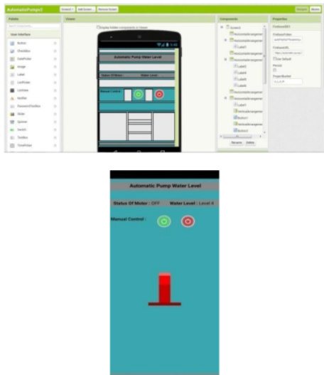
Gambar 14. Perancangan aplikasi
