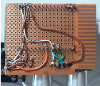
Gambar 9. Rangkaian NodeMCU ESP8266
