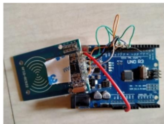
Gambar 6. Perakitan Alat
