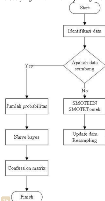
Gambar 2. flowchart metode yang diusulkan
