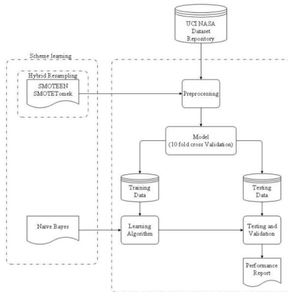
Gambar 1. kerangka kerja metode yang diusulkan
