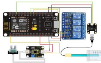
Gambar 3 Rangkaian Keseluruhan
